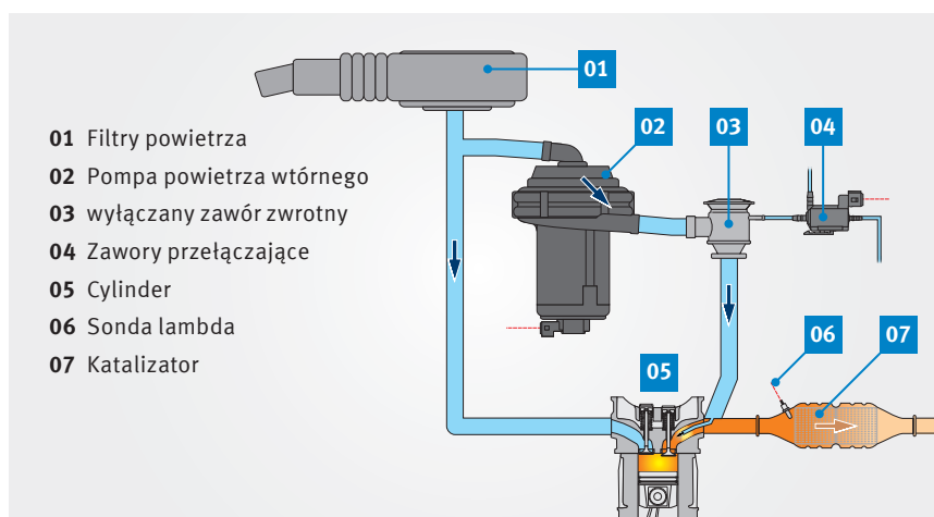
Zasada wdmuchiwania powietrza wtórnego (zasterowanie pneumatyczne)
